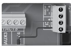
Sonde Chlore Libre ① rouge ④ noir
