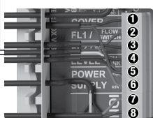
③ negro ⑤ marrón ⑥ azul
