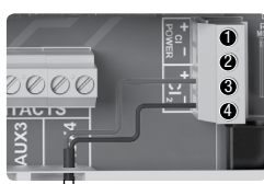
Freies Chlor Sonde ③ rot ④ schwarz
